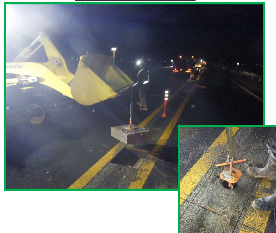
既設舗装版撤去状況(機械)
