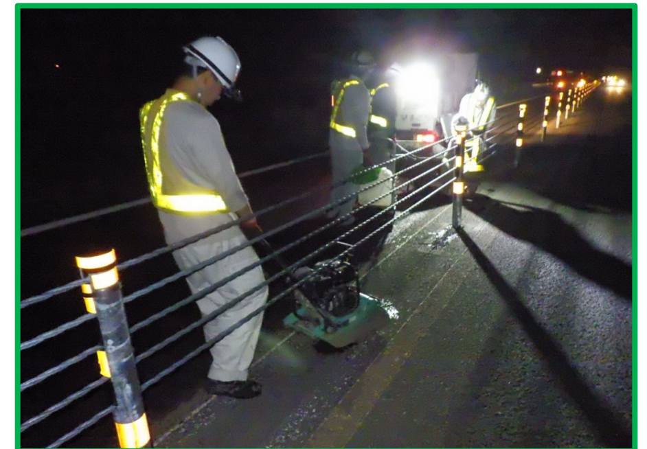
常温合材転圧状況
