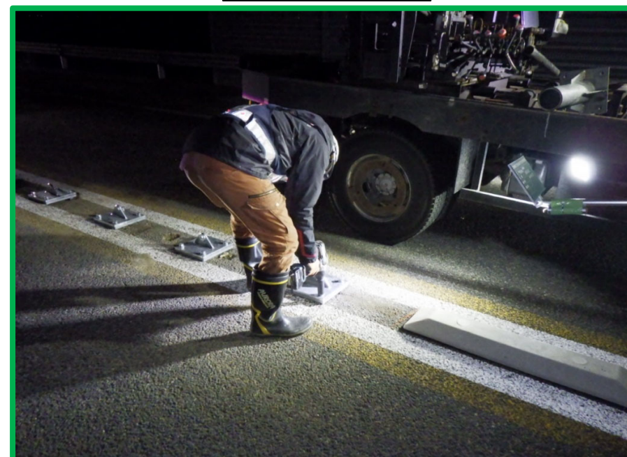
頭部金具取付状況
