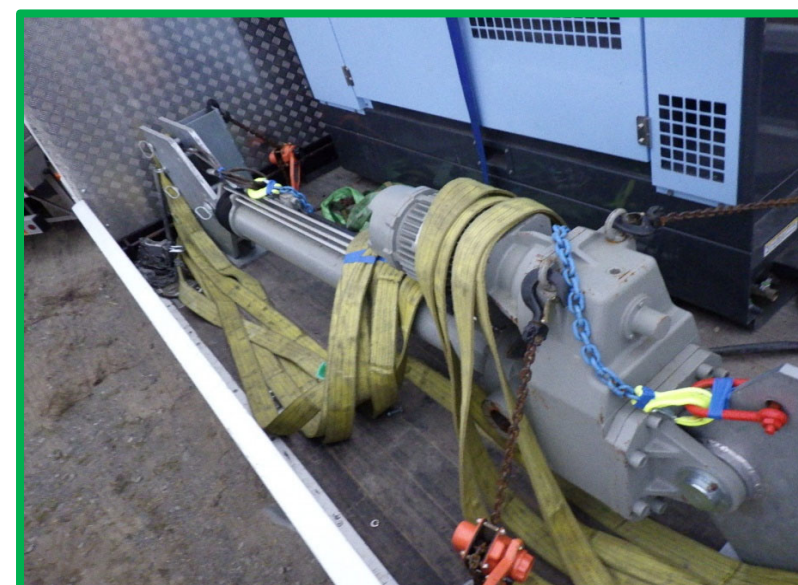
パワーシリンダー(中間ターンバックル施工用)
