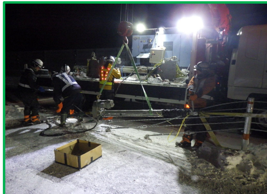
ワイヤーロープ 仮緊張状況(パワーシリンダー使用)
