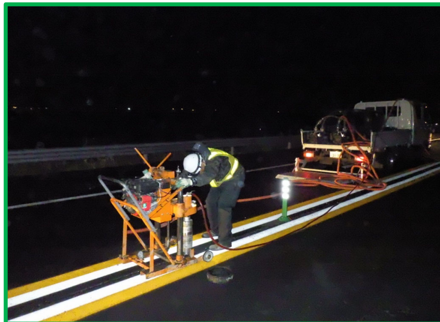
Asコア削孔状況(エンジン式)
