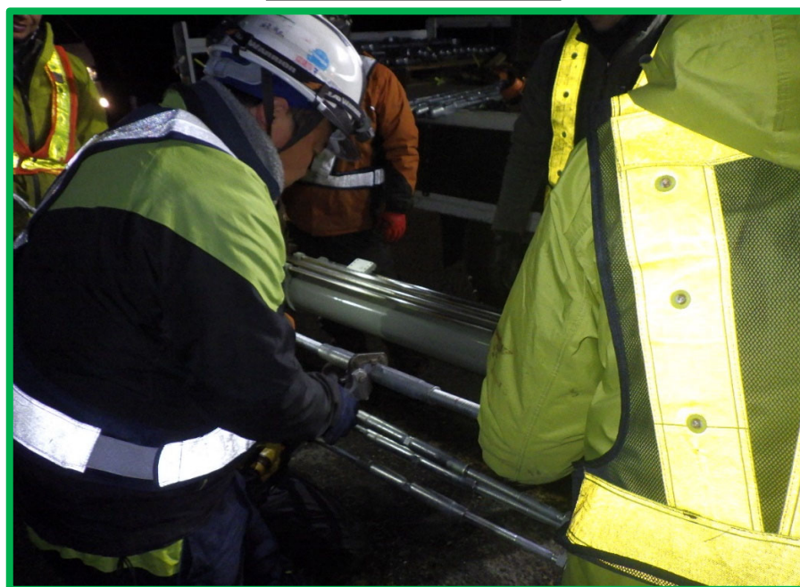
ターナックル締付け状況
