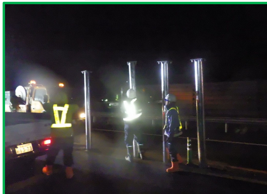
端末鋼管杭建込み状況
