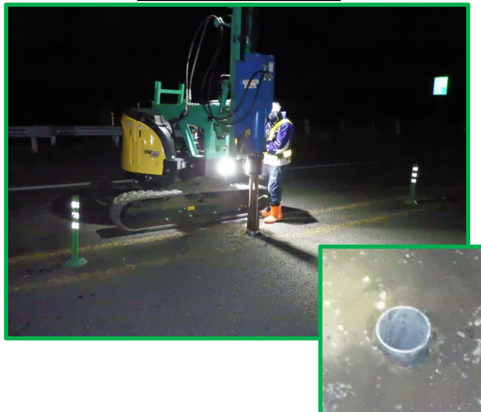
スリーブ鋼管打込み状況
